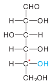
D-glukóza
